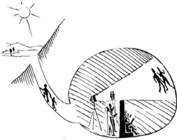
„Höhlengleichnis“
