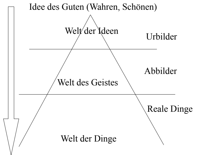
„Ideenlehre“
